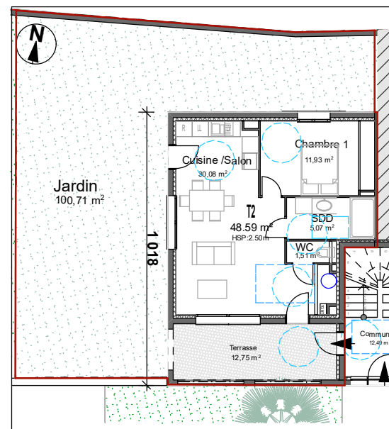
RDC / APPT 1 / Ech: 1/200
